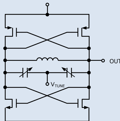
図 4 LC VCO
