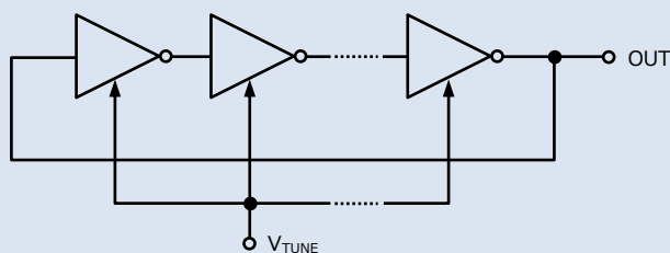
図 3 Ring VCO
