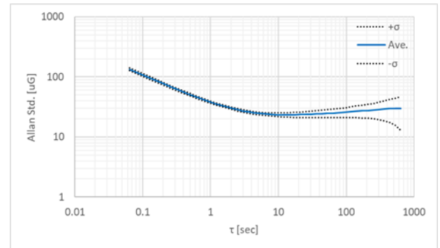
加速度センサーのルートラン分散特性
