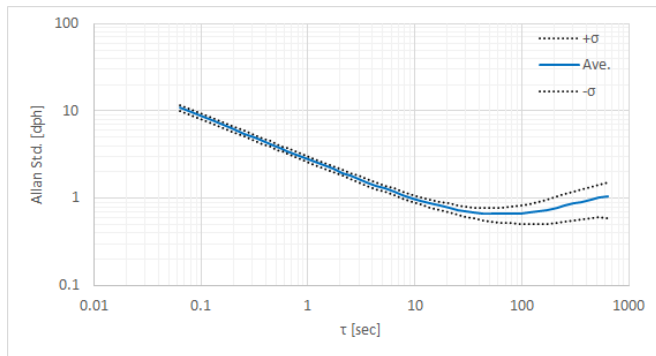
ジャイロセンサーのルートラン分散特性
