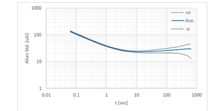
加速度センサーのルートアラン分散特性
