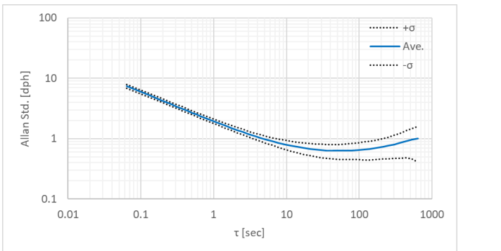
ジャイロセンサーのルートアラン分散特性
