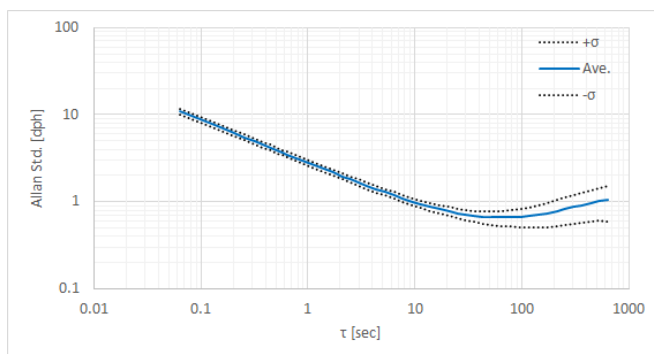
ジャイロセンサーのルートアラン分散特性
